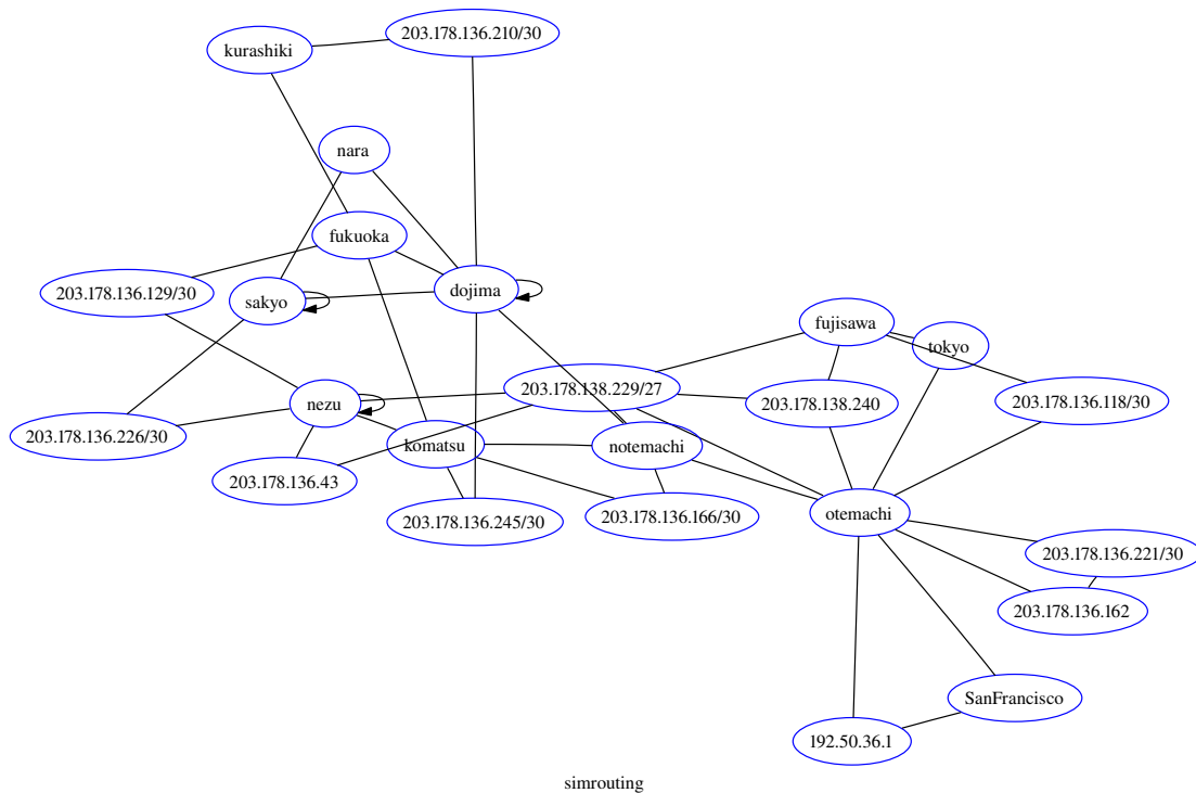
図 1: WIDE Project ネットワークトポロジ (2006/12/24)
